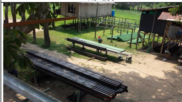
Foto 3: Perfiles C metálicos para los puentes colgantes
