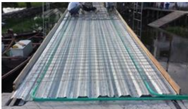
Fotografías 1 y 2. Steel deck que conforma la formaleta de la estructura metálica para fundida de la placa en concreto
